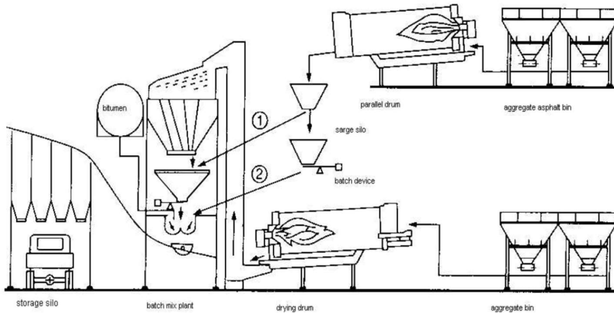
Chargemenger met paralleltrommel
